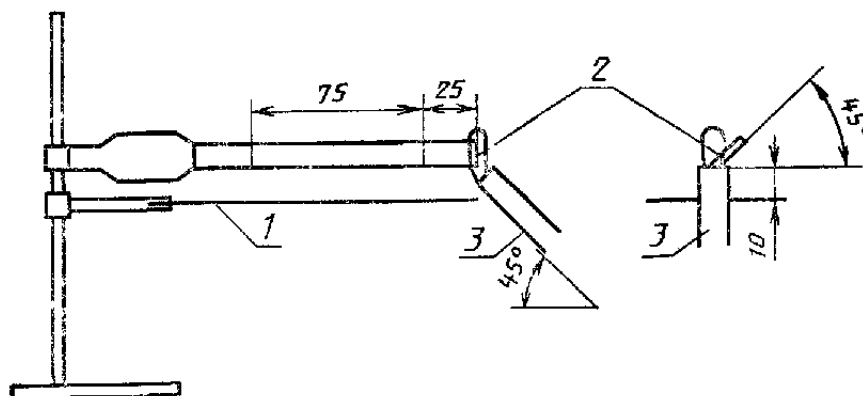
1 - металлическая (проволочная) сетка; 2 - образец; 3 - горелка
